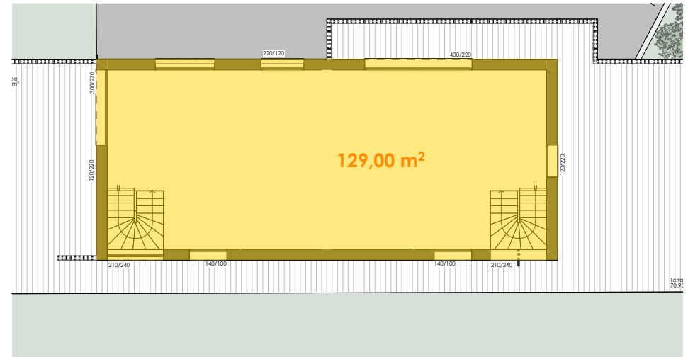
1/200 PLAN REZ-DE-CHAUSSEE
