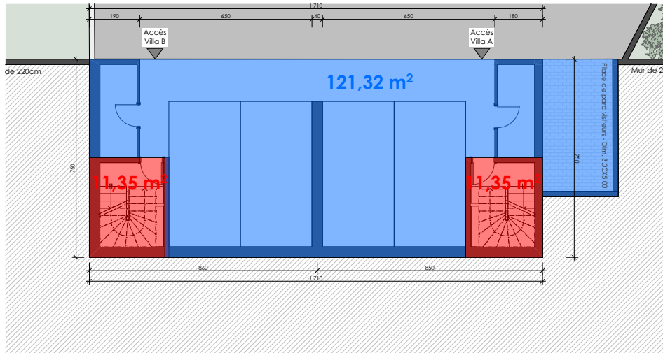
1/200 PLAN SOUS-SOL
